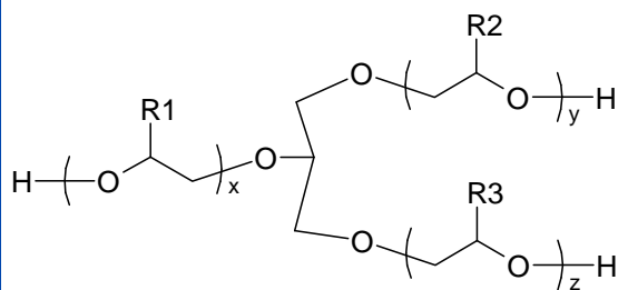
Kuva 4: Yksi kuvaus glyserolin, etyleenioksidin ja propeeniksiidin reaktiotuotteen yleisestä rakenteesta (x, y ja z ovat kokonaislukuja, R1, R2 ja R3 ovat vetyatomeja tai metyyliryhmiä).
