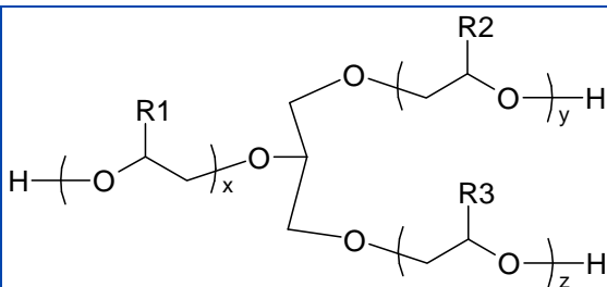
Figura 4: Representación de la estructura general del producto de la reacción del glicerol, el óxido de etileno y el óxido de propileno («x», «y» y «z» son números enteros, R1, R2 y R3 son átomos H o grupos de metilo).
