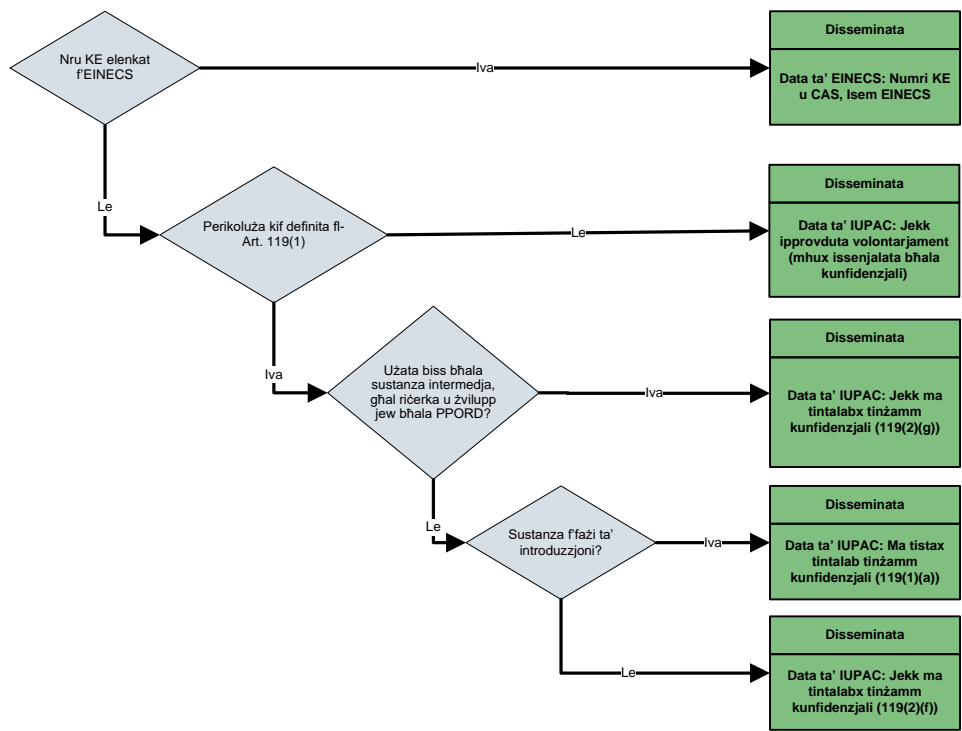
Figura 4: Flowchart biex jiġi ddeterminat jekk id-data IUPAC ta' sustanza rreġistrata hijiex ser tiġi ppubblikata
