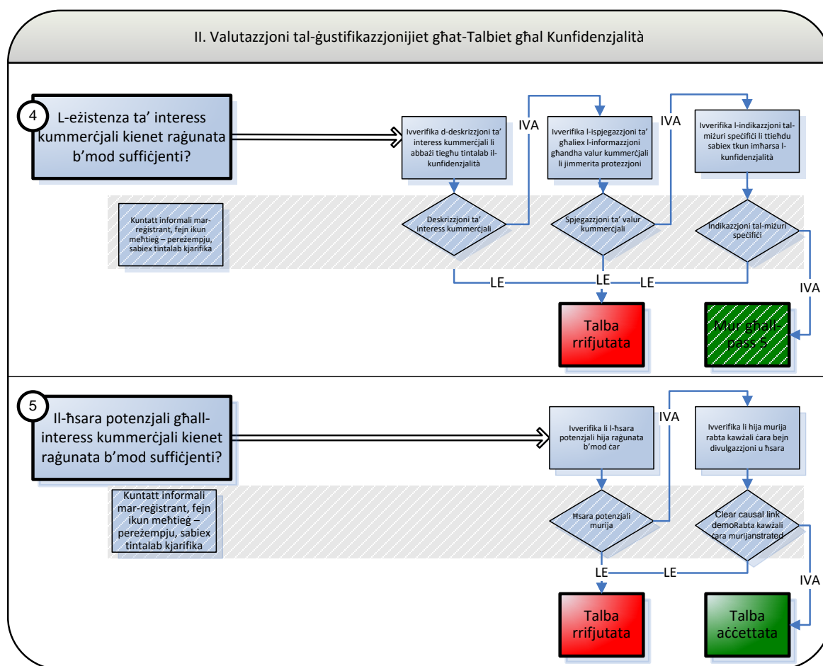
Figura 14: Fluss tax-xogħol għall-Valutazzjoni ta' Ġustifikazzjonijiet għal Talbiet għal Kunfidenzjalità
